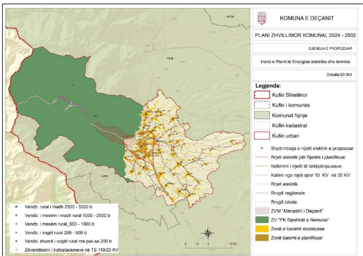
Harta 52 Rrjeti energjetik në Komunën e Deçanit – planifikimi
