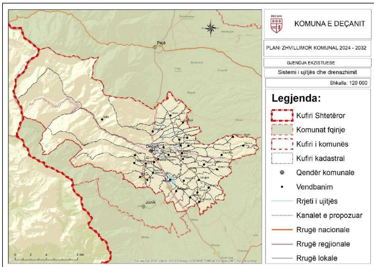
Harta 12 Sistemi i ujitjes dhe drenazhimit
