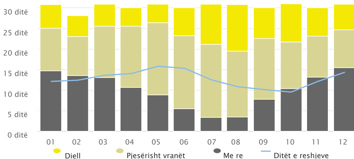
Grafiku 8 Ditët me diell, me re, vranësira dhe reshje
