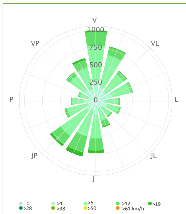
Grafiku 18 Trëndafili i erërave
