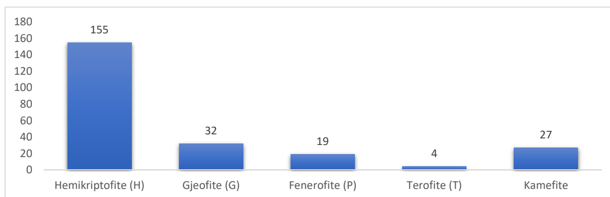
Grafiku 15 Taksonet e përhapjes të bimëve sipas ndarjes se Raunkierit (format jetësore sipas Raunkierit)
