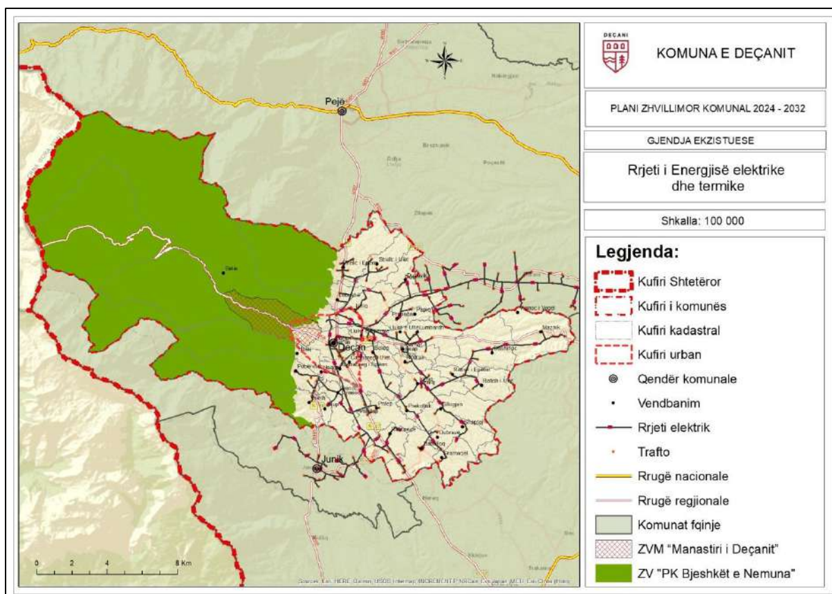
Harta 13 Rrjeti elektrik
