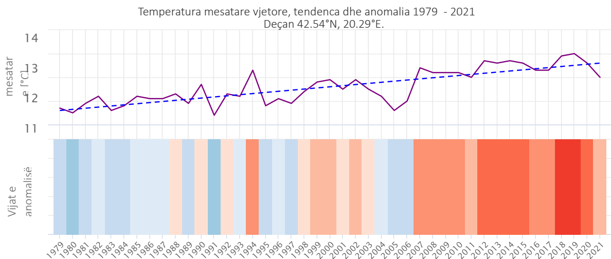
Grafiku 10 Temperaturat mesatare vjetore, tendencat dhe anomalitë
