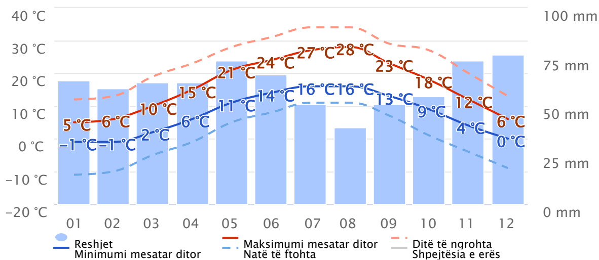
Grafiku 11 Temperaturat mesatare vjetore dhe reshjet
