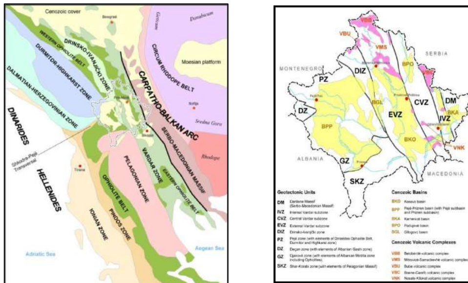
Figura 12 Njësitë gjeotektonike të Ballkanit Qendror dhe në Kosovë
